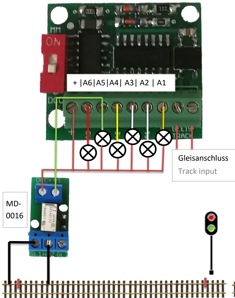
Ohne MFB-Modul mit Relais (Art-0016)
